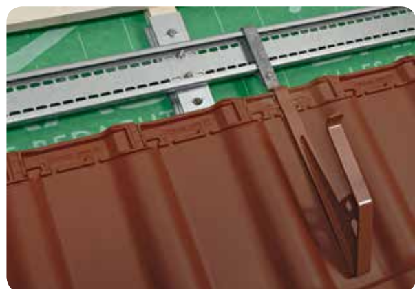
Beispiel: DivoDämm EasyFix SHD mit Sicherheitsdachhaken 3R
