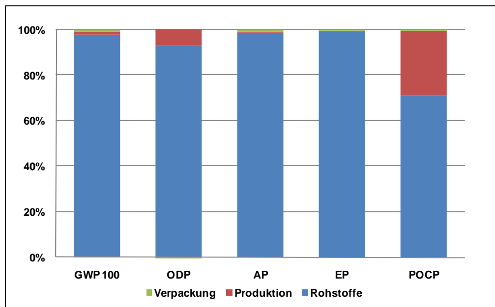
Abbildung 8-3: Relative Beiträge zu den Umweltwirkungen für die Herstellung von 1 m 3 PUR/PIR Alu
