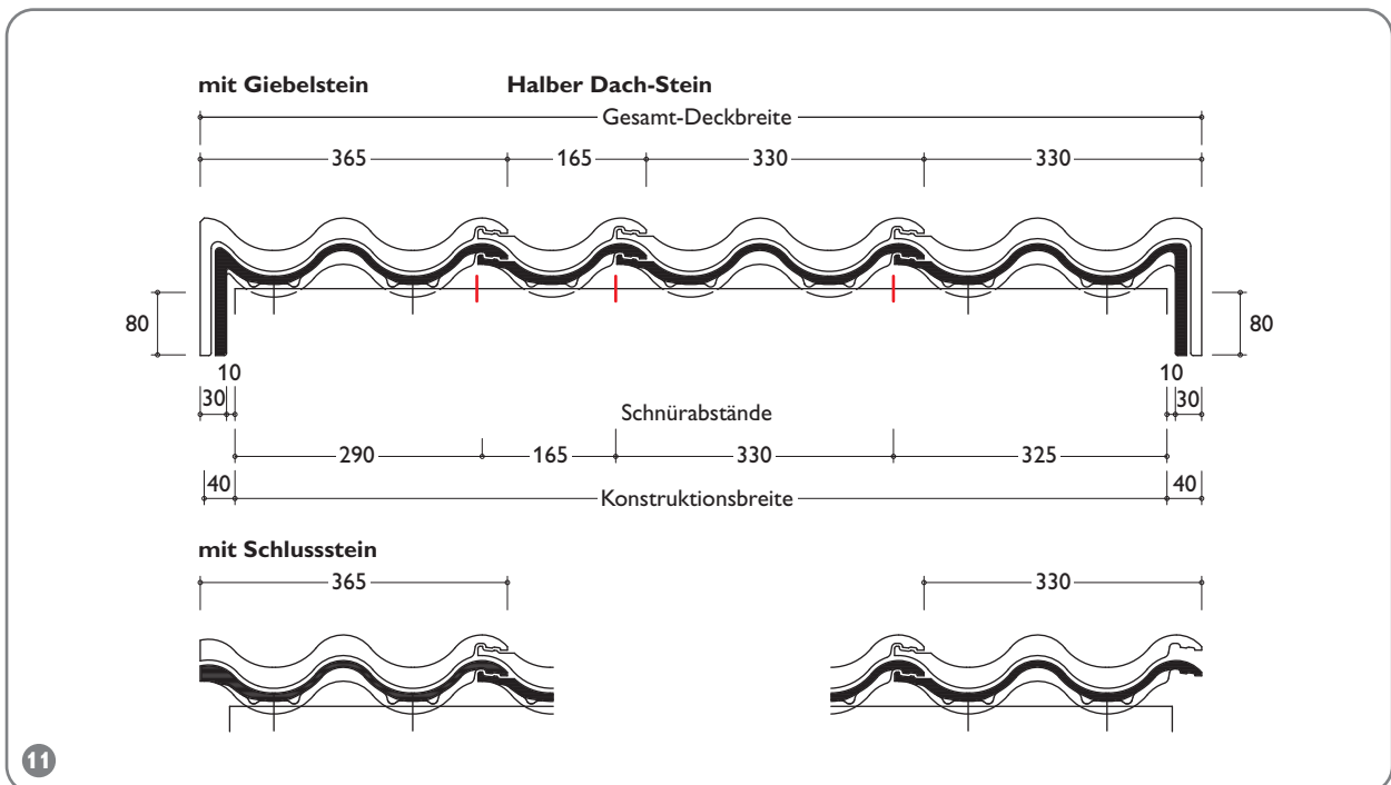
Konstruktionsbreite = jeweils Schnürabstand Ortgang rechts + Dach-Steine + Halber Dach-Stein + Ortgang links Tabelle 15
