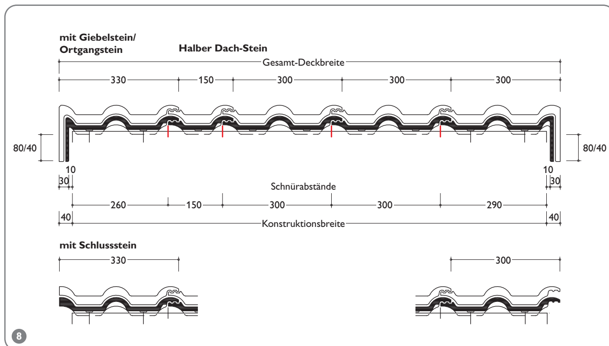
Konstruktionsbreite = jeweils Schnürabstand Ortgang rechts + Dach-Steine + Halber Dach-Stein + Ortgang links Tabelle 11
