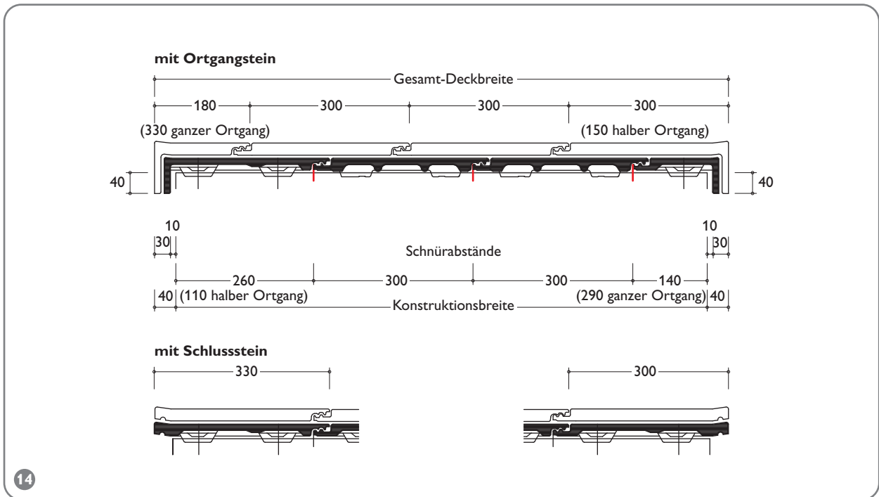
Konstruktionsbreite = jeweils Schnürabstand Ortgang rechts + Dach-Steine + Halber Dach-Stein + Ortgang links Tabelle 19
